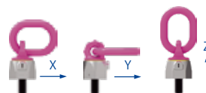
■吊り方と荷重方向
